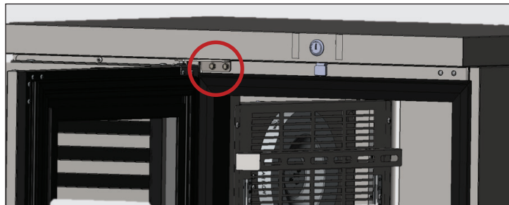
Abb. 1. Die Befestigungsschrauben der oberen Scharnierwinkel entfernen.
