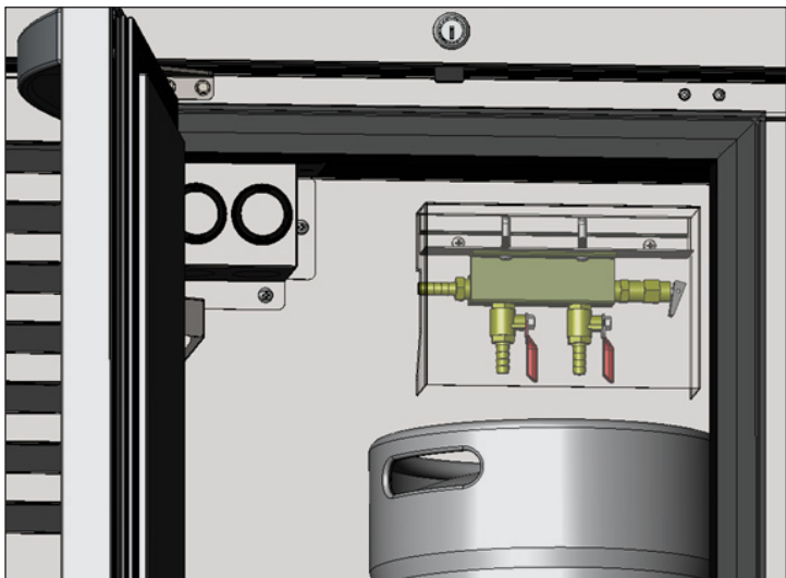
Abb. 2. 2-Wege-Verteiler.
