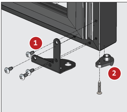
Fig. 7a. Ensemble de composants de la charnière inférieure.
