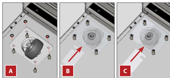
Fig. 7. Pose des cales de roulette par paires.
