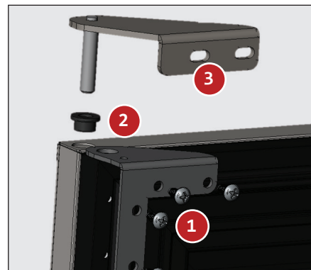
Fig. 7b. Ensemble de composants de charnière supérieure.
