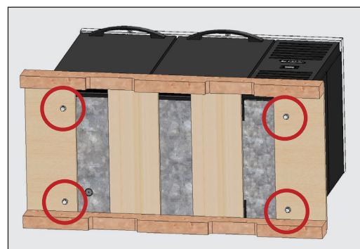
Fig. 2. Emplacements des boulons de transport.
