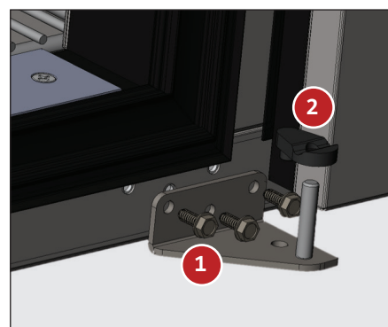
Fig. 9. Installez l'axe de la charnière inférieure dans son nouvel emplacement.
