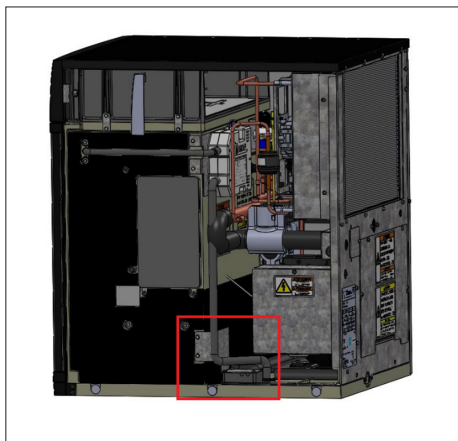
Рис. 1. Место установки датчика уровня льда.
