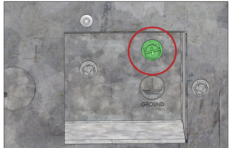
Рис. 3. Выполнить электрические соединения внутри соединительной коробки льдогенератора. Обязательно использовать устройства для снятия механического напряжения. Обязательно использовать зеленый винт заземления при выполнении электрических соединений.
