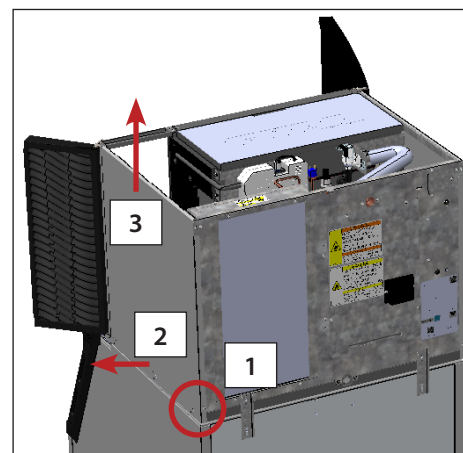
Рис. 3. Вывернуть винт, снять панель с язычков крепления, затем поднять и снять.
