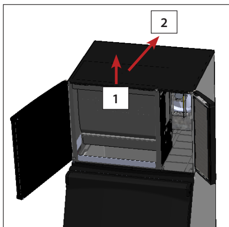
Рис. 2. Поднять передний край, сдвинуть верхнюю панель назад, затем поднять и снять ее.
