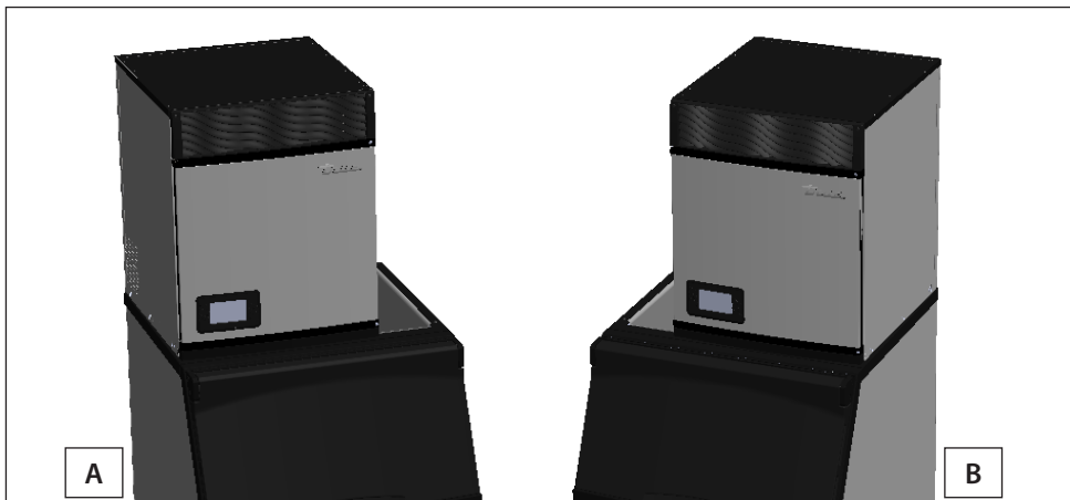
Рис. 3. 22-дюймовый льдогенератор, установленный слева (А) и справа (В) на 30-дюймовом контейнере с помощью переходного устройства.
