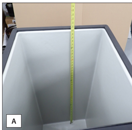
Рис. 2. Перед установкой льдогенератора обязательно измерить глубину контейнера (А) или диспенсера (В) для настройки датчика уровня льда.
