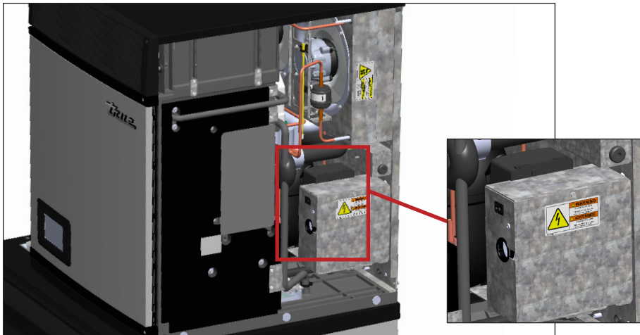
Рис. 2. Расположение кулисного выключателя. Кулисный переключатель отключает питание от платы управления и переднего дисплея; он НЕ ОТКЛЮЧАЕТ питание всего устройства.
