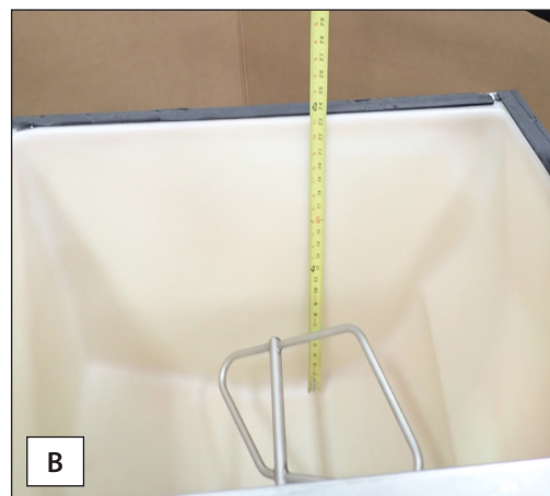
Рис. 2. Перед установкой льдогенератора обязательно измерить глубину контейнера (А) или диспенсера (В) для настройки датчика уровня льда.
