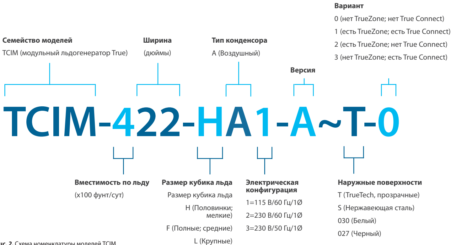
Рис. 2. Схема номенклатуры моделей TCIM.
