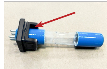
Rys. 4. Wgłębienie na gumowej uszczelce.
