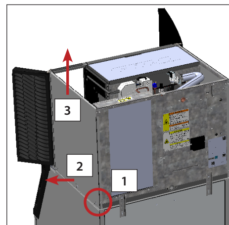
Rys. 3. Wykręcić śrubę, odkleić od podkładek i zdjąć, unosząc.
