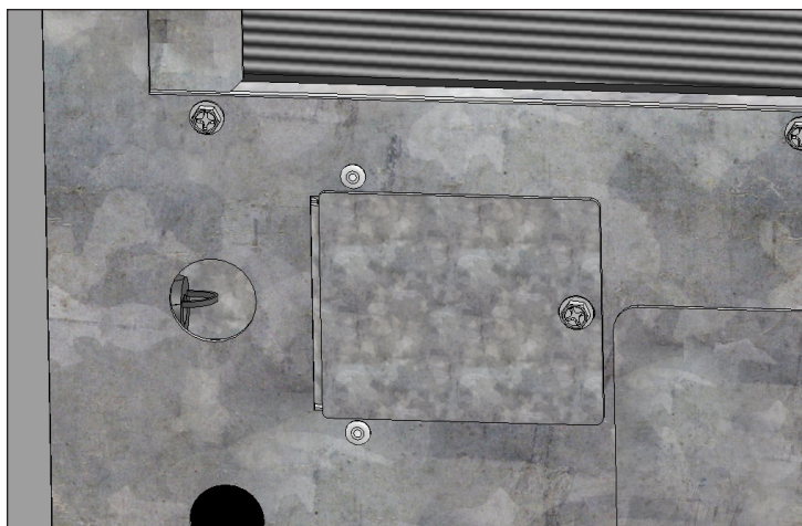
Rys. 3. Wykonanie przyłącza elektrycznego w skrzynce przyłączeniowej kostkarki do lodu. Używać przepustów kablowych. Wykonując przyłącza elektryczne, zawsze należy wykorzystywać zieloną śrubę zaciskową uziemienia.
