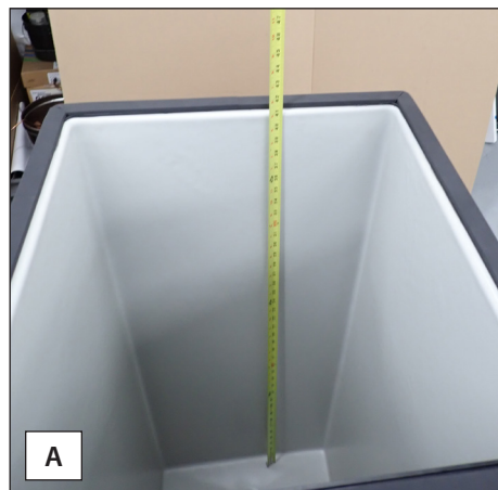
Rys. 2. Zawsze przed instalacją kostkarki do lodu wykonać pomiary zasobnika (A) lub dystrybutora (B) na potrzeby czujnika poziomu kostek lodu.
