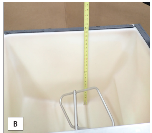
Rys. 2. Zawsze przed instalacją kostkarki do lodu wykonać pomiary zasobnika (A) lub dystrybutora (B) na potrzeby czujnika poziomu kostek lodu.
