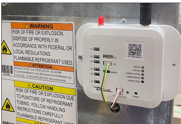
Rys. 2. Wiązka modemu podłączona do modemu. Zielony/żółty do TEC; brązowy/biały do ZASILANIA.
