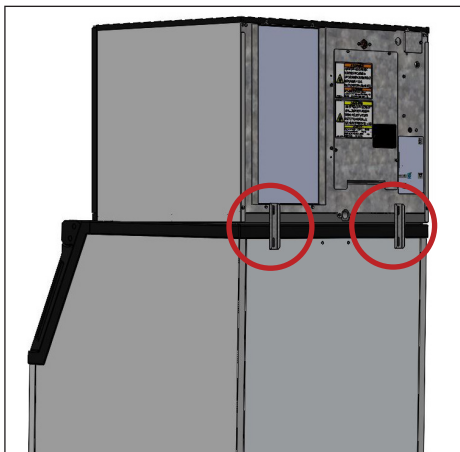
Rys. 1. Zamontować wsporniki zasobnika.
