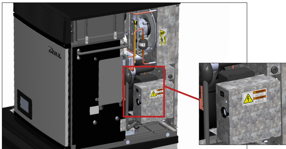
Rys. 2. Położenie przełącznika kołyskowego. Przełącznik kołyskowy odłącza zasilanie tablicy sterowania i wyświetlacza przedniego, lecz NIE ODŁĄCZA zasilania całego urządzenia.
