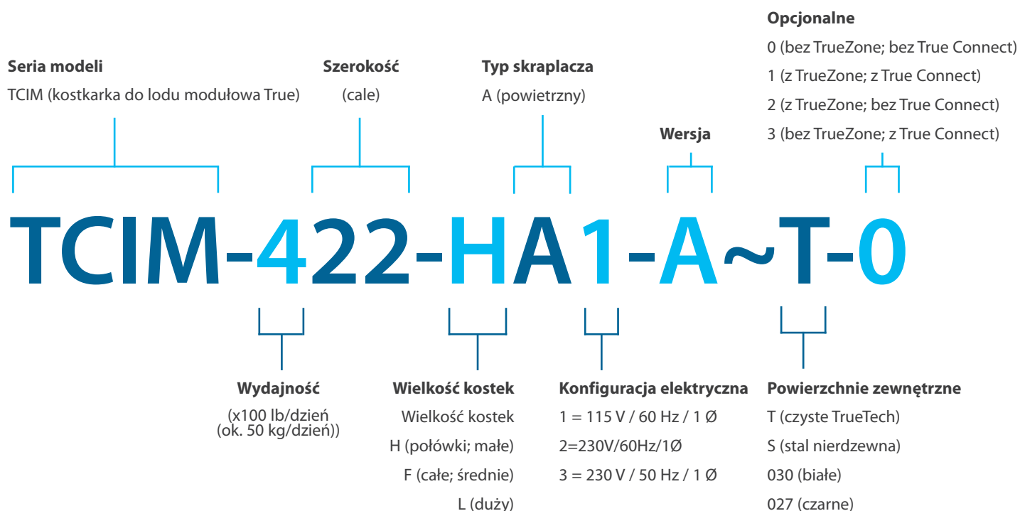
Rys. 2. Schemat komponentów numeru modelu TCIM.
